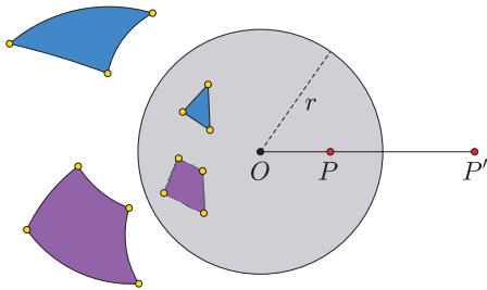
1. ábra. Az ábrán egy pont és két sokszög inverz képe van. Látható, hogy az inverz geometria nem kezeli jól a háromszögeket, négyszögeket, ezért érdemesebb csak a pontok, egyenesek és körök képeivel foglalkozni
