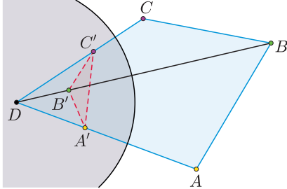
4. ábra. Ábra a Ptolemaiosz-egyenlőtlenséghez
